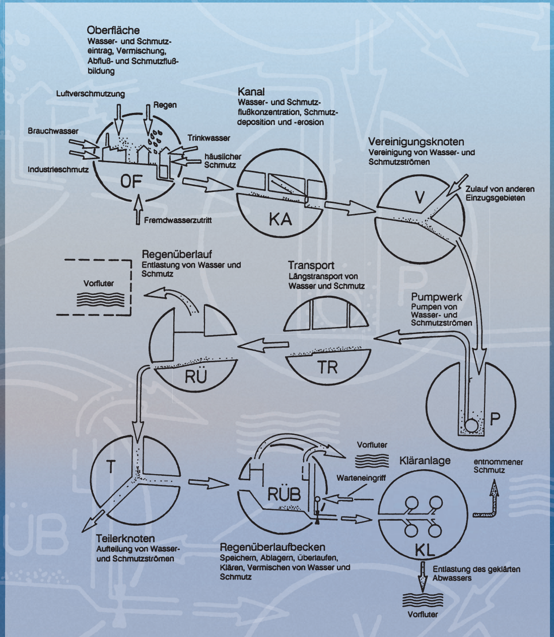
Darstellung der Modellbausteine zum UFT-eigenen Schmutzfrachtsimulationsmodell ASMI aus dem Jahr 1982 von Dr. Brombach. Heute wird die Schmutzfrachtberechnung mit dem Modell KOSIM aus dem Hause itwh durchgeführt, und statt „Vorfluter“ sagt man „Gewässer“.
