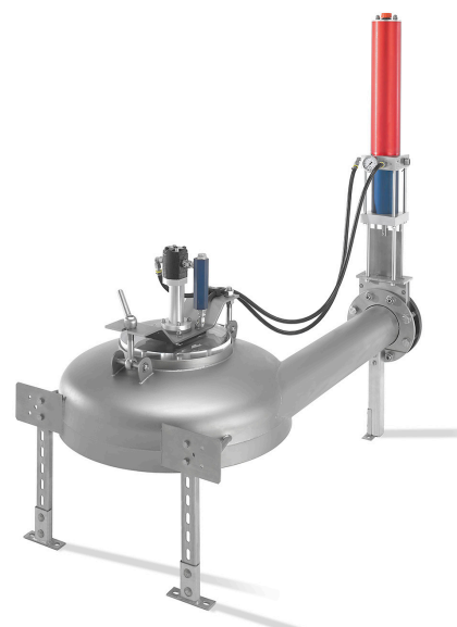
Bild 6: Einbaufertige Turbo-Wirbeldrossel UFT-FluidTurbo DN 150
